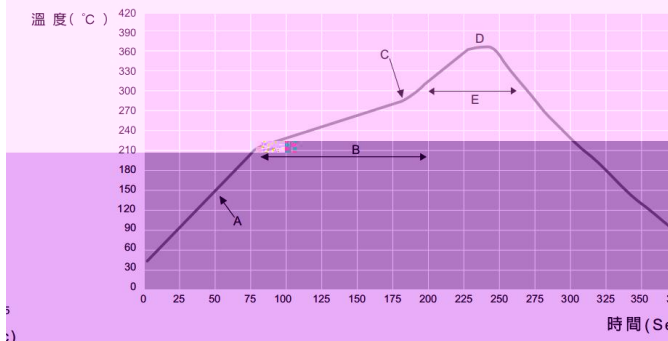
高 铅 锡 膏 熔 温 曲 线 图
